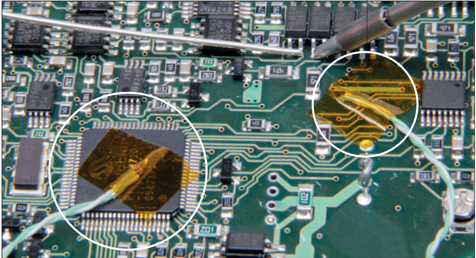
Hilfstermoelement (TC)
